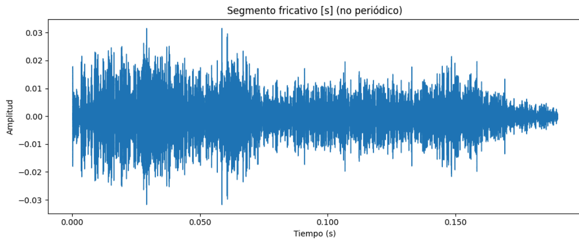
Figura 5. Segmento fricativo [s] de "lapachos" rápido
